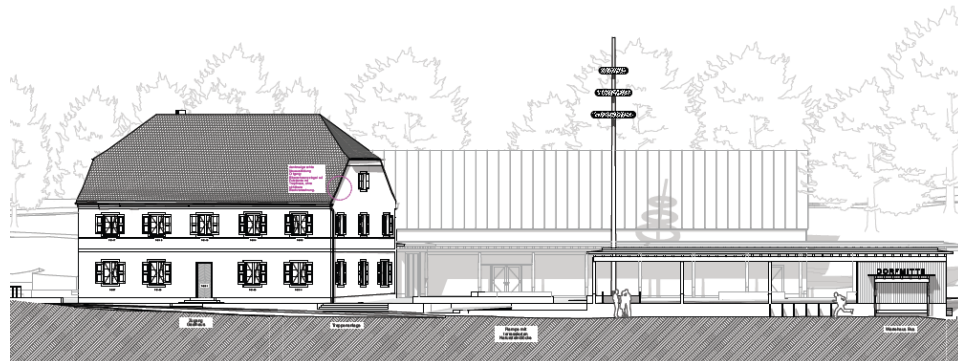
Anzicht Süd (Nümburger Straße)
