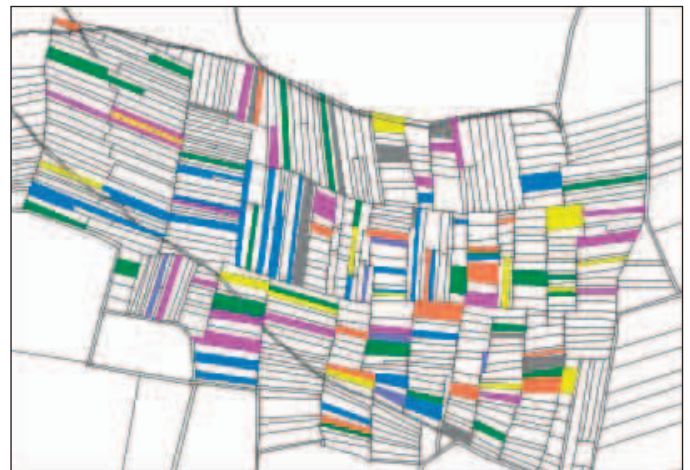
Waldneuordnung: vorher
